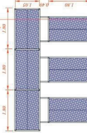
SEZIONE A-A
