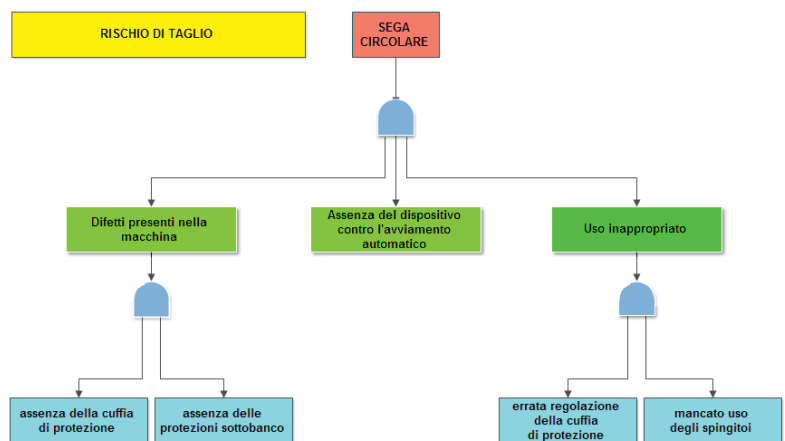
ESEMPIO DI ALBERO DELLE CAUSE - RISCHIO DI TAGLIO: SEGA CIRCOLARE
