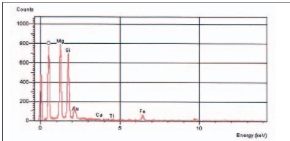
Fig. 6 – Spettro EDX crisotilo
