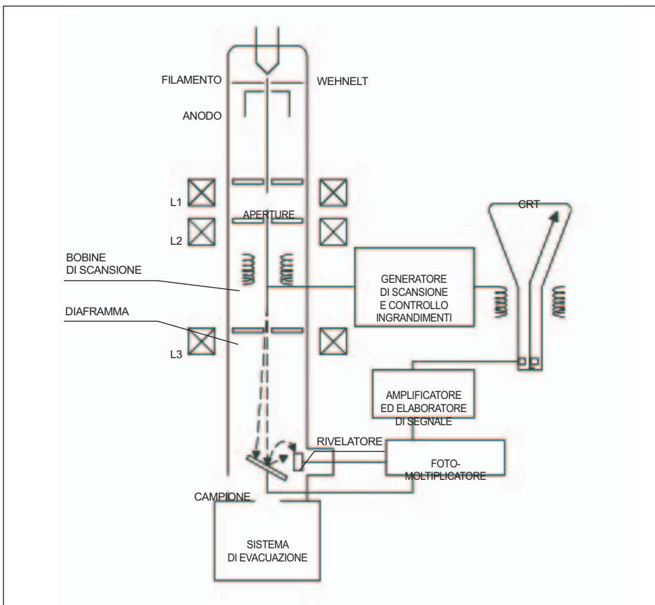
Fig. 4 - Schema a blocchi di un tipico SEM con colonna elettronica costituita da tre lenti elettromagnetiche L1, L2, L3. La figura riporta una configurazione adatta a fornire immagini di morfologia superficiale.
